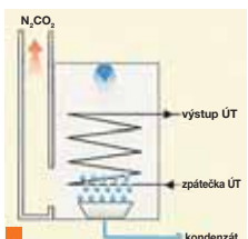
Princip spalování kondenzačního kotle
